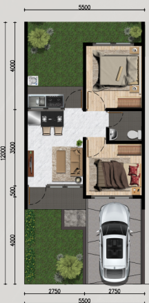
Tipe A 5,5 x 12 m FLAT
